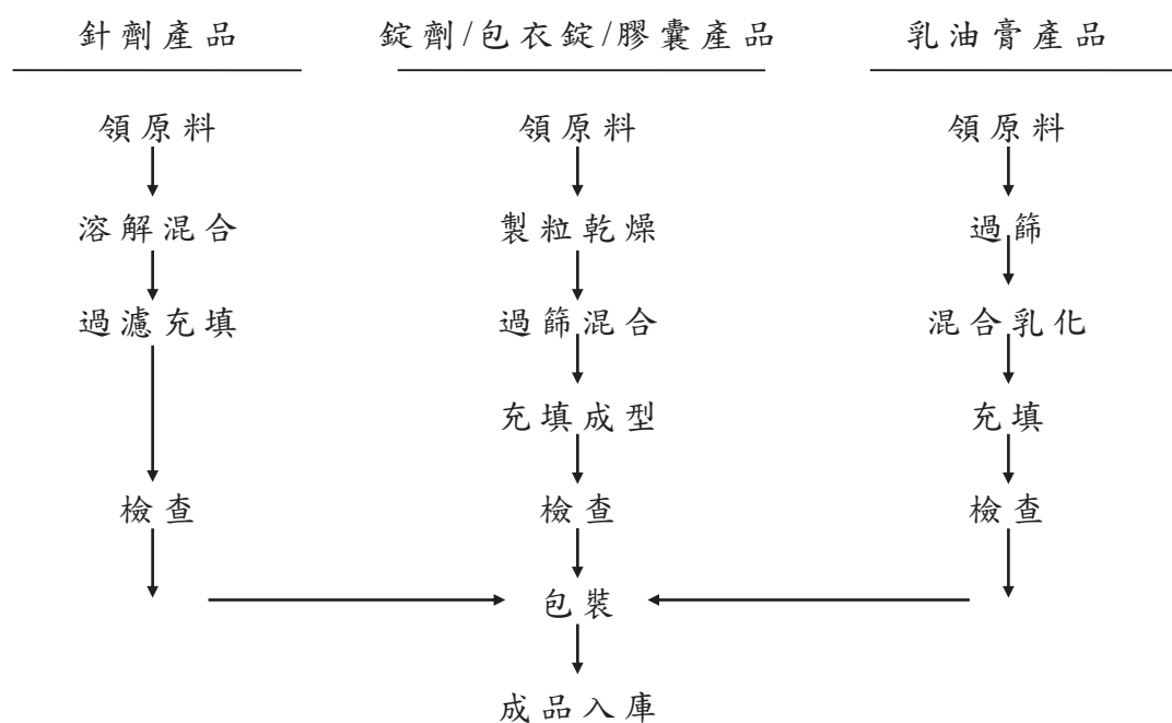
生產流程圖
