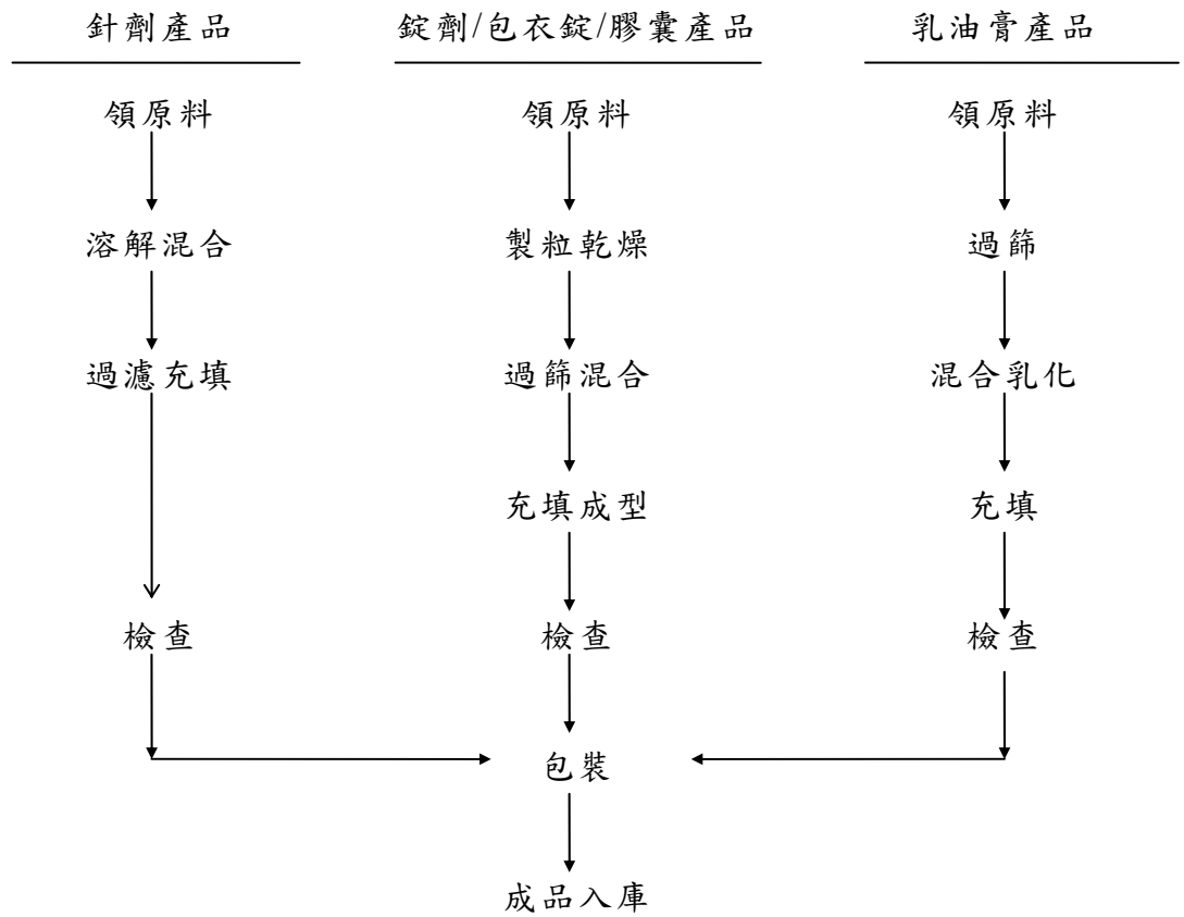
生產流程圖
